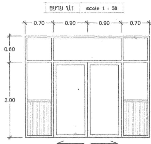
ป.1 ประตูบานเลื่อนกระจกกรอบอลูมิเนียม ขนาด 0.90X2.00 ม. คู่
