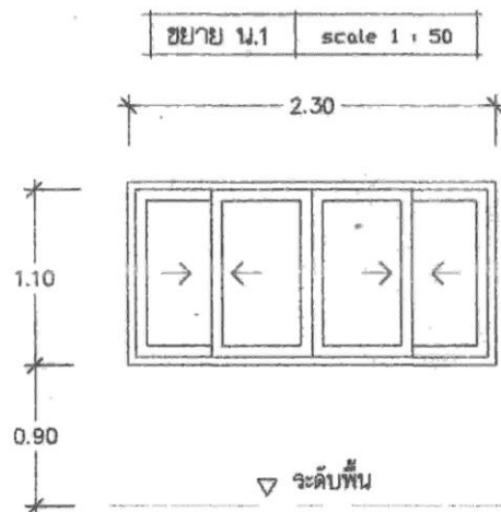
4.9 หน้าต่างบานเลื่อนกรอบบานและวงกบอลูมิเนียม
