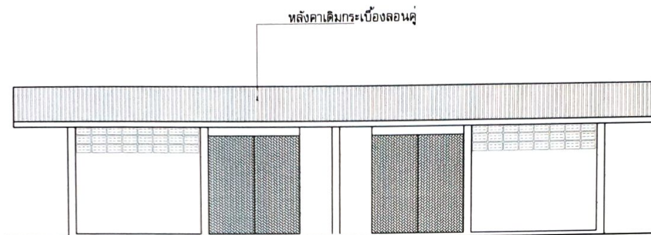
รูปด้านหน้าเดิม มาตราส่วน 1 : 100
