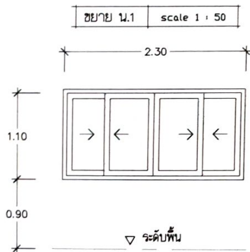
น.5 หน้าต่างบานเลื่อนกรอบบานและวงกบอลูมิเนียม
